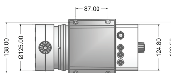
CORPS DE POMPE « T »
