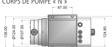
CORPS DE POMPE « N »
