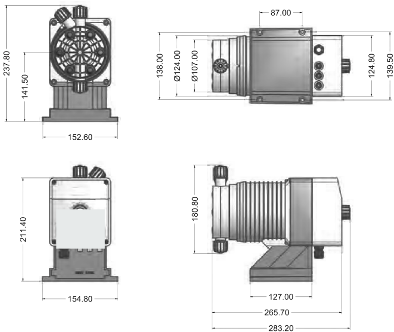
Fig. 16. Dimensions de la pompe corps de pompe modèle S ou T
