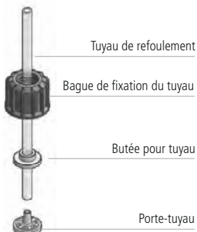
Fig. 5. Assemblage du tuyau de refoulement/corps de pompe.
