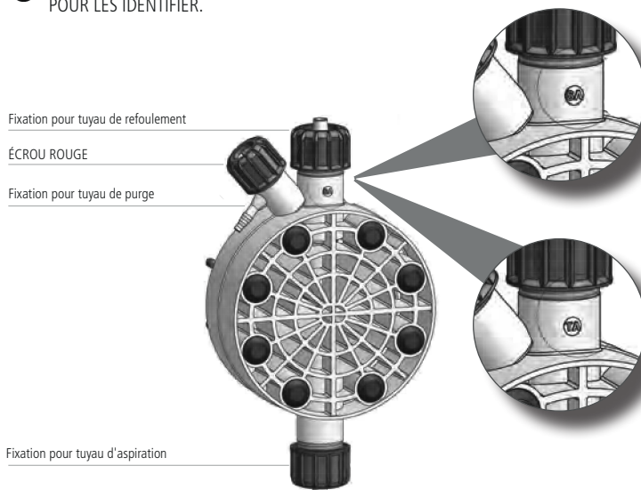
Fig. 8. Description du corps de pompe auto-vidangeant modèles: SA, TA
