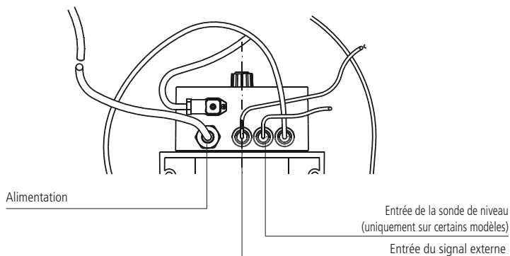
Fig. 10. Raccordements de la pompe.
