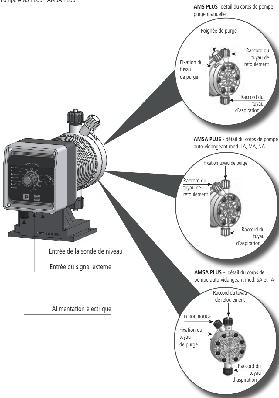
Fig. 1. Pompe AMS PLUS - AMSA PLUS
