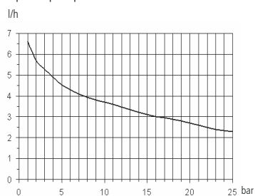
Fig. 14. Courbes de débit des modèles auto-vidangeants
