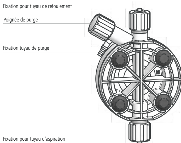
Fig. 6. Description du corps de pompe avec purge manuelle (AMS PLUS).
