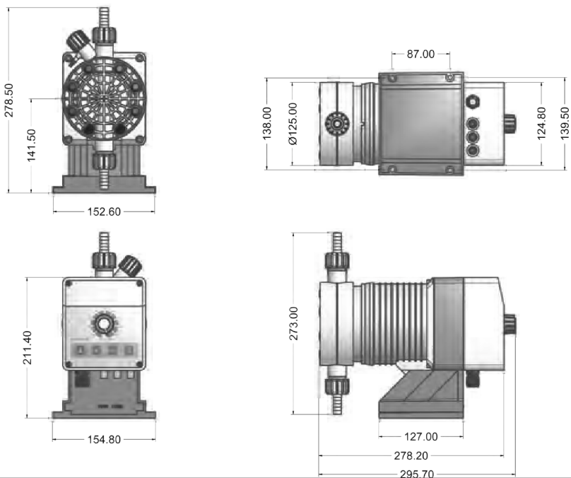
Fig. 16. Dimensions de la pompe corps de pompe modèle S ou T
