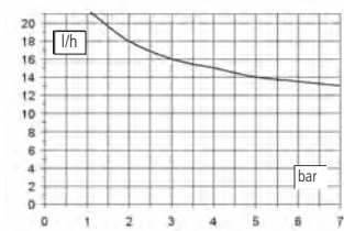
Corps de pompe NA
