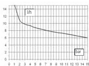
Corps de pompe MA
