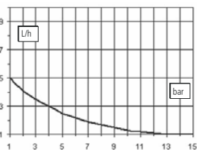
Corps de pompe KA
