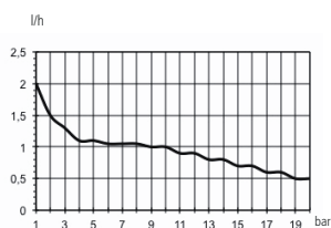
Fig. 12. Courbes de débit VAPO
