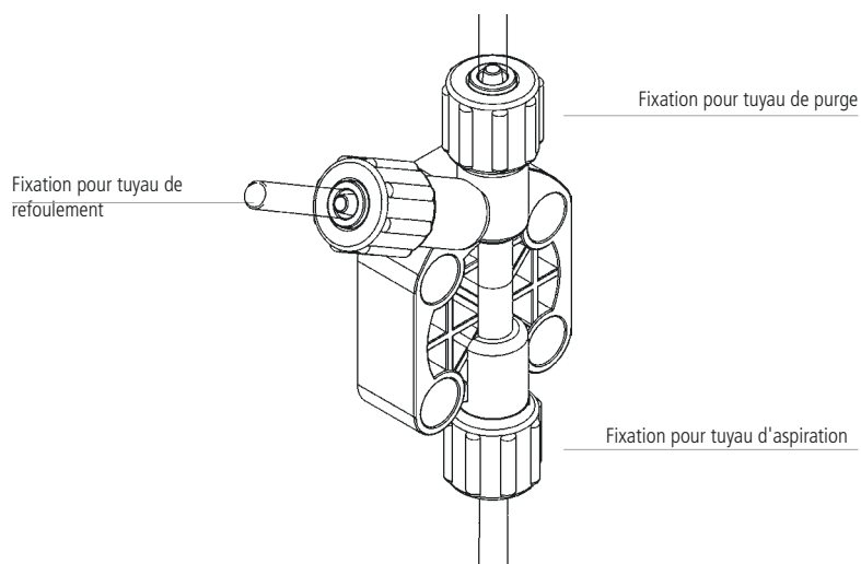
Fig. 7. Description du corps de pompe auto-vidangeant
