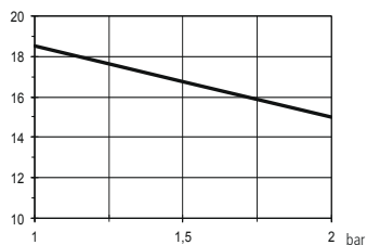
0215: l/h 15 bar 2 Corps de pompe modèle K l/h
