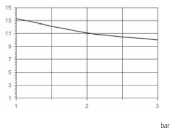
0116: l/h 16 bar 1 Corps de pompe modèle K l/h
