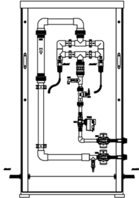
Abb. 2 - Aufbau (Rückseite)
