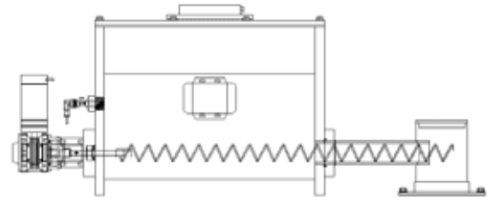
Abb. 2 - Zuführschnecke
