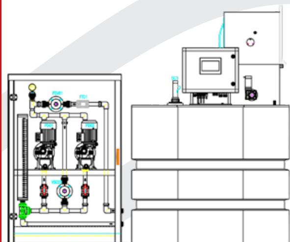
Abb. 2 - Aufbau PermaDos SE + Skid Safety Box
