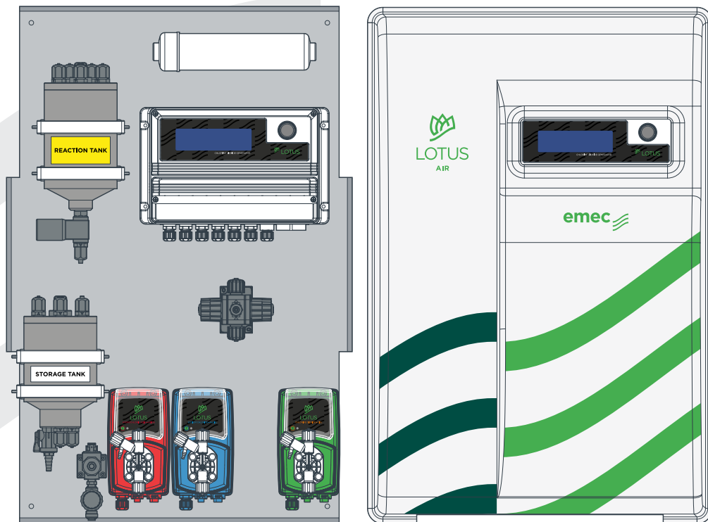
Abb. 1 - Aufbau
