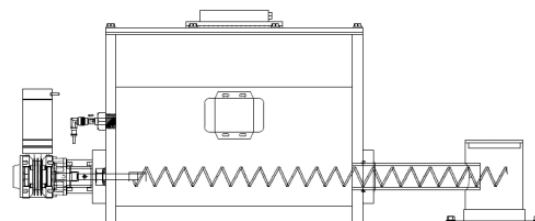
Fig. 2 - Vis d'alimentation
