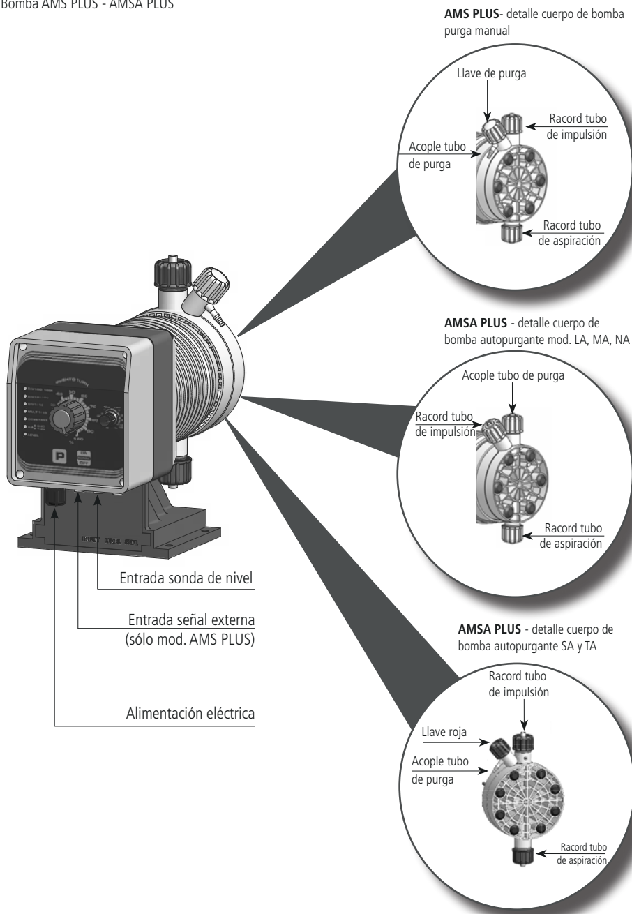
Fig. 2. Bomba AMS PLUS - AMSA PLUS
