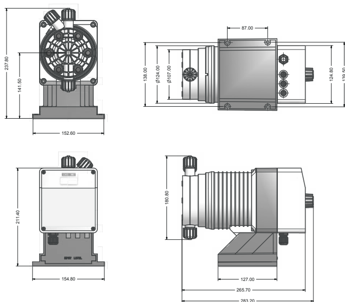
Fig. 18. Dimensiones bomba con cabezal mod. S o T
