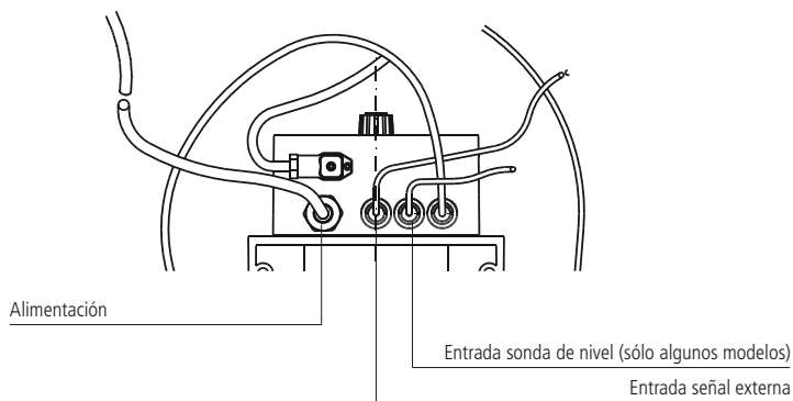
Fig. 11. Conexión de la bomba.
