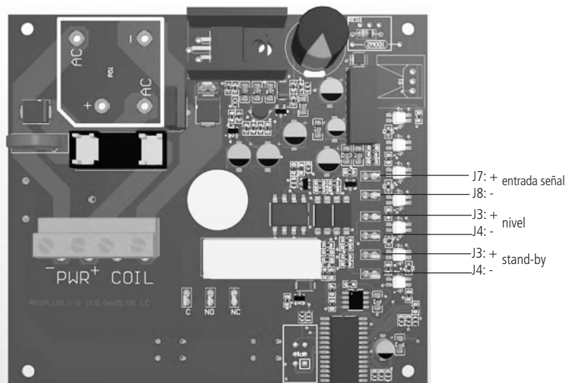
Fig. 14. Esquema circuito AMS PLUS 12 VDC
