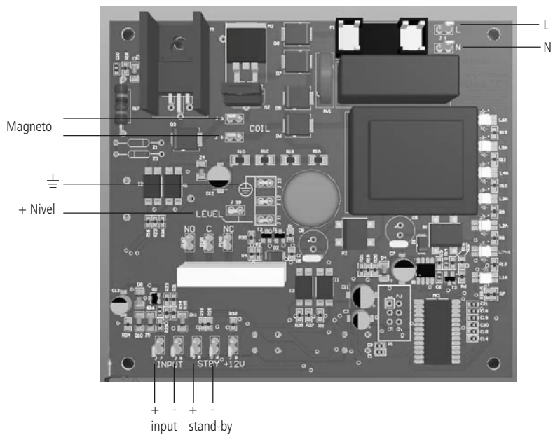
Fig. 13. Esquema circuito AMS PLUS 230/115 VAC
