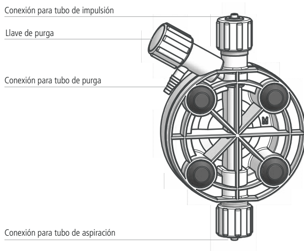
Fig. 7. Descripción cuerpo de bomba con purga manual (AMS PLUS)
