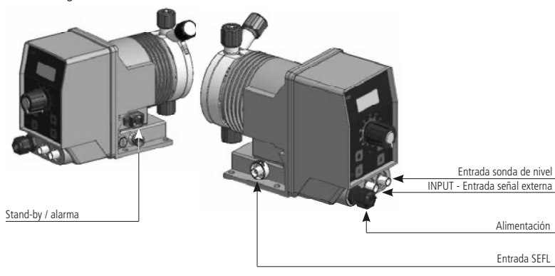
Fig. 13. Conexionado de la bomba
