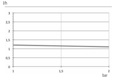
0301: 1 l/h 3 bar Cabezal mod. I
