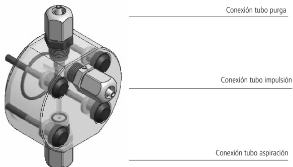
Fig. 10. Cabezal en PMMA autopurgante (bomba KMSA MF).
