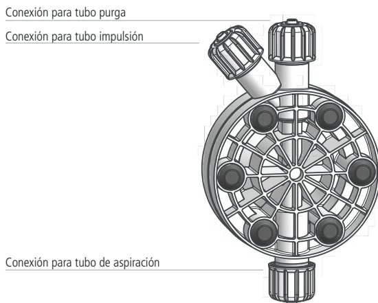
Fig. 7. Cabezal autopurgante mod.: SA, TA (bomba TA).
