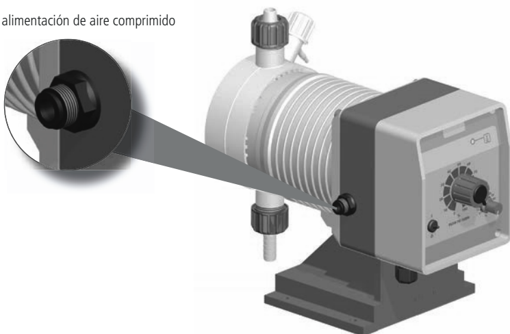
Figura 2. Bomba dosificadora AMS AC
