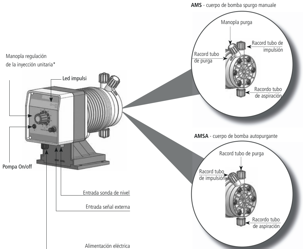
Figura 1. Bomba dosificadora AMS - AMSA
