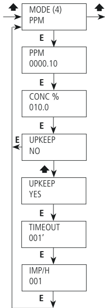
Fig. 19. Menú PPM.
