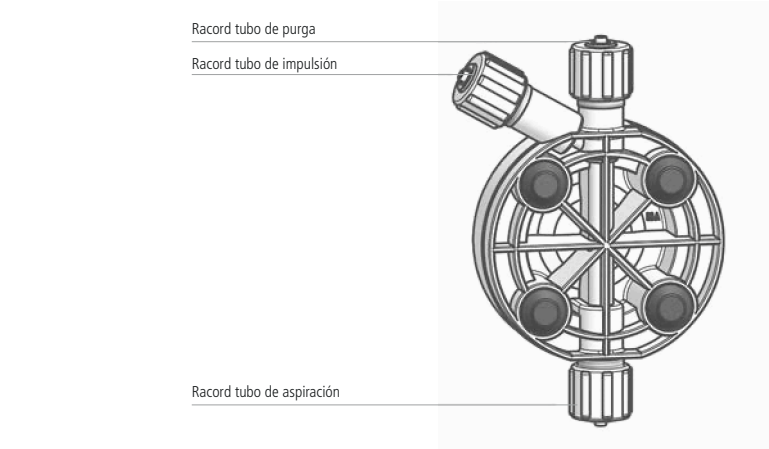
Fig. 11. Descripción cuerpo de bomba autopurgante modelos: SA, TA (bomba AMSA MF).
