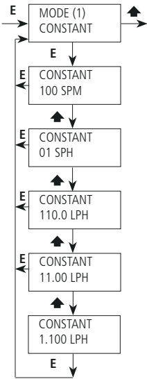
Fig. 16. Menú Constant.
