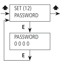
Fig. 43. Menú Password.
