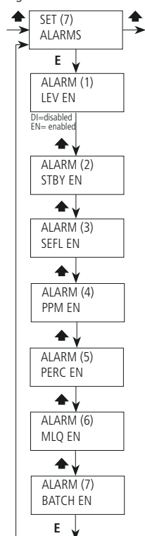
Fig. 37. Menú Alarmas.
