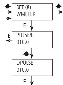
Fig. 38. Menú Wmeter.
