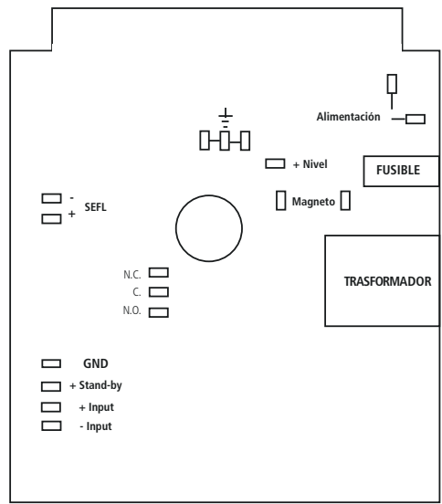
Fig. 46. Esquema circuito AMS MF
