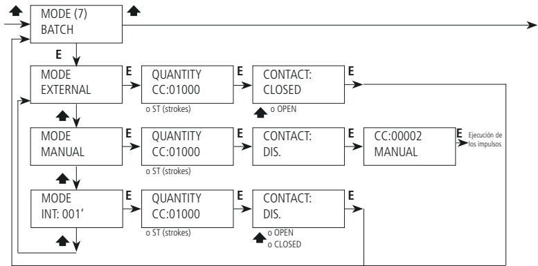
Fig. 22. Menú BATCH
