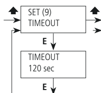
Fig. 39. Menú Timeout.
