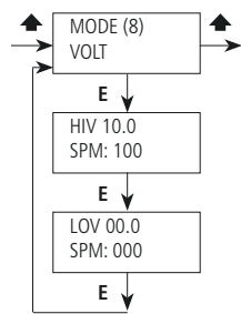
Fig. 28. Menú VOLT
