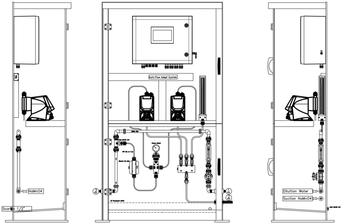
Fig. 1 - Panneau d'instrumentation
