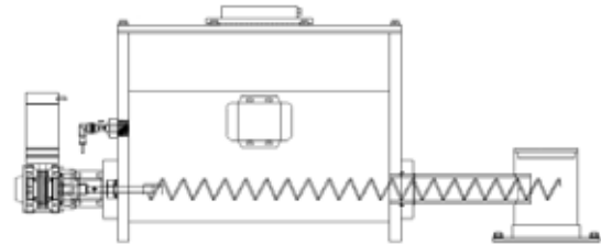
Fig. 2 - Vis d'alimentation
