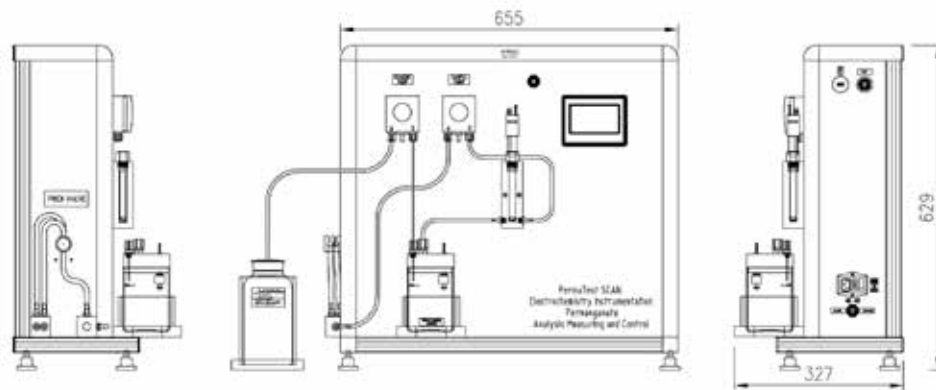
Fig. 1 - Panneau d'instrumentation
