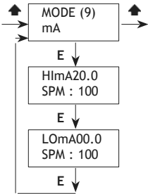
Fig. 24. Menu mA
