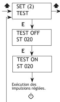
Fig. 26. Menu TEST
