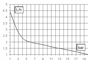
Corps de pompe J
