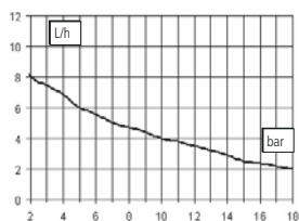
Corps de pompe KA
