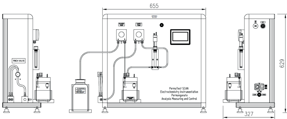
Fig. 1 - Pannello strumentazione
