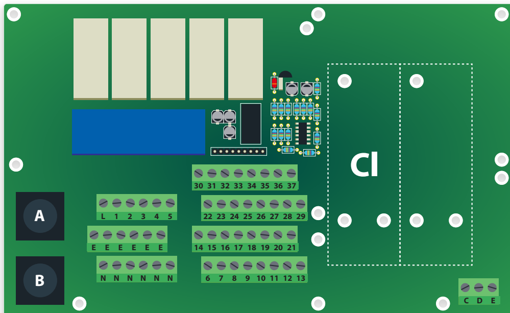
*example mainboard
