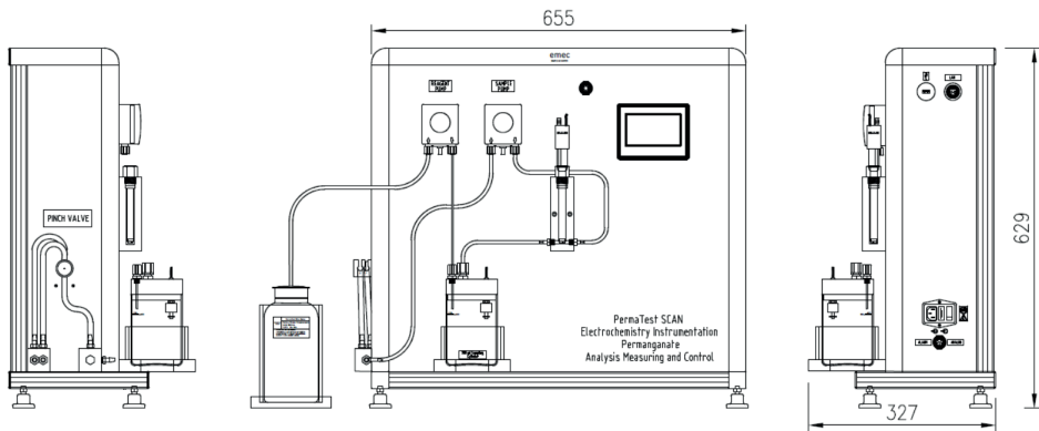
Abb. 1 - Aufbau
