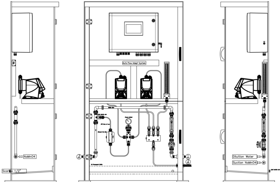
Fig. 1 - Pannello strumentazione
