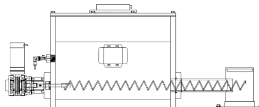
Fig. 2 - Coclea di alimentazione
