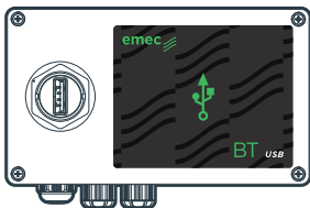
BT USB Dispositivo para guardar registros en USB. IP65.
