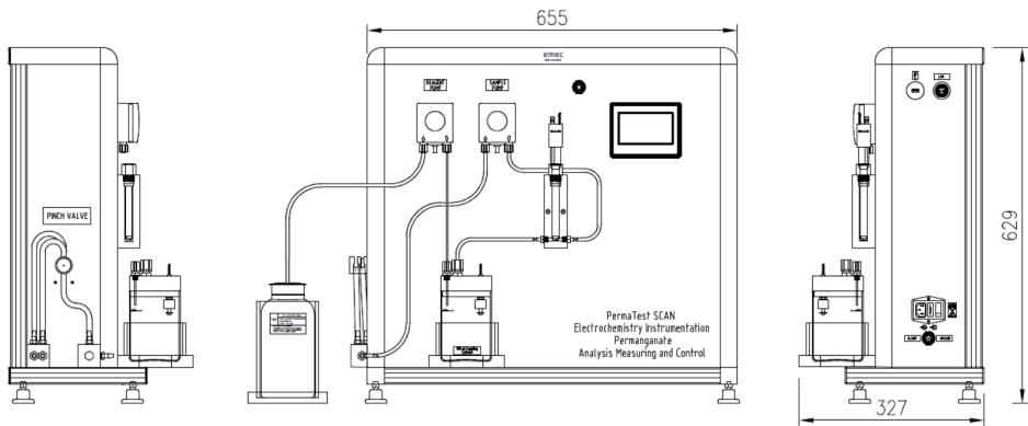
Fig. 1 - Pannello strumentazione
