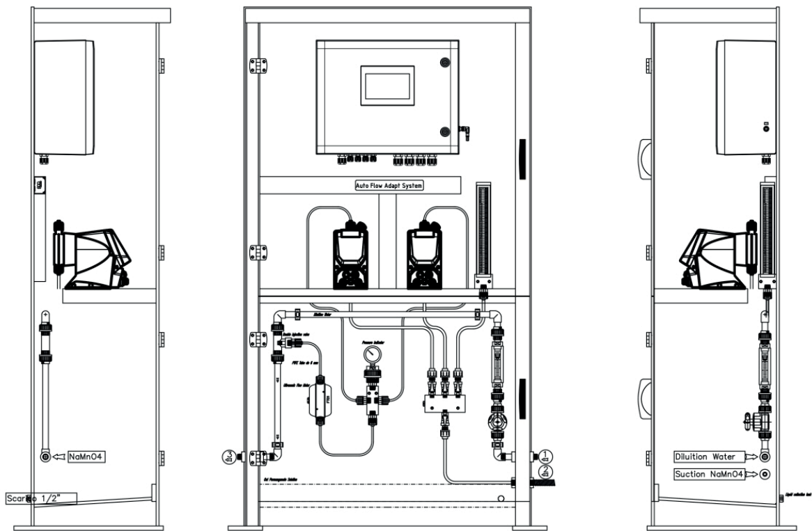
Fig. 1 - Panneau d'instrumentation
