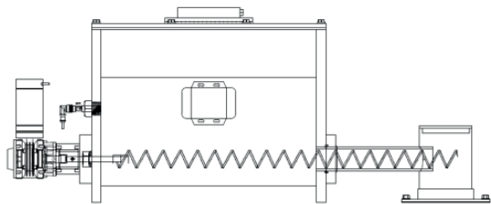
Fig. 2 - Vis d'alimentation
