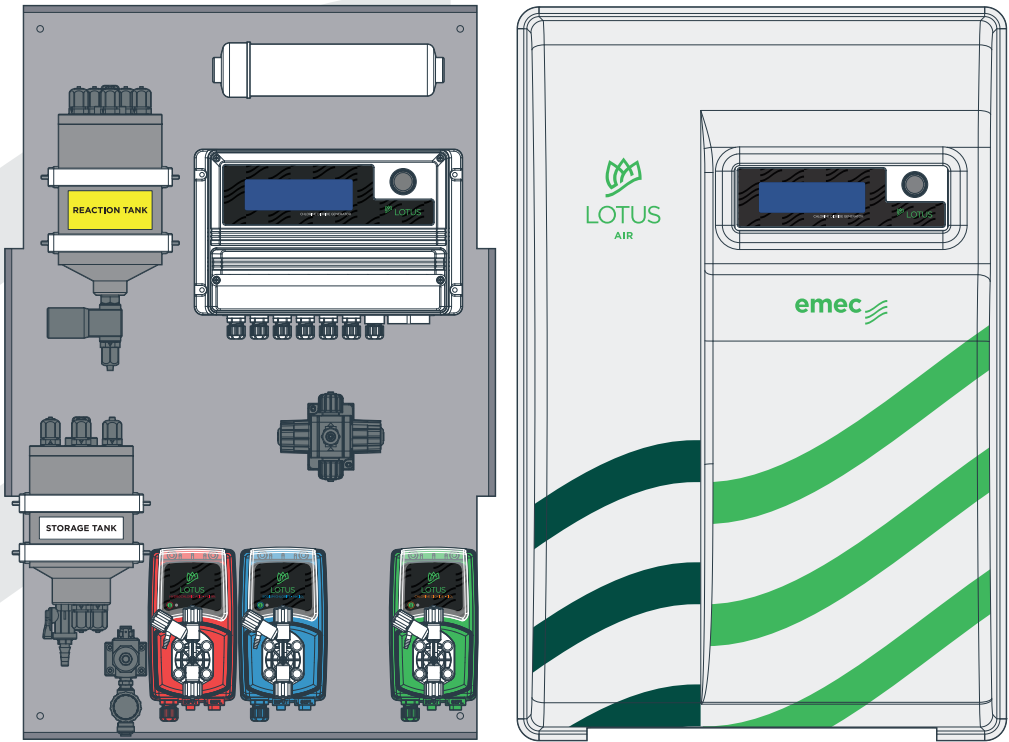
Fig. 1 - Capot et intérieur de l'appareil
