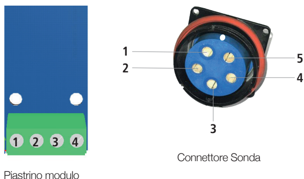
Piastrino modulo
