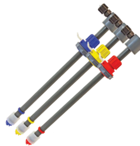
LASP Sauglansen komplett mit Füllstandssonde für Behälter bis zu 1000 Liter.
