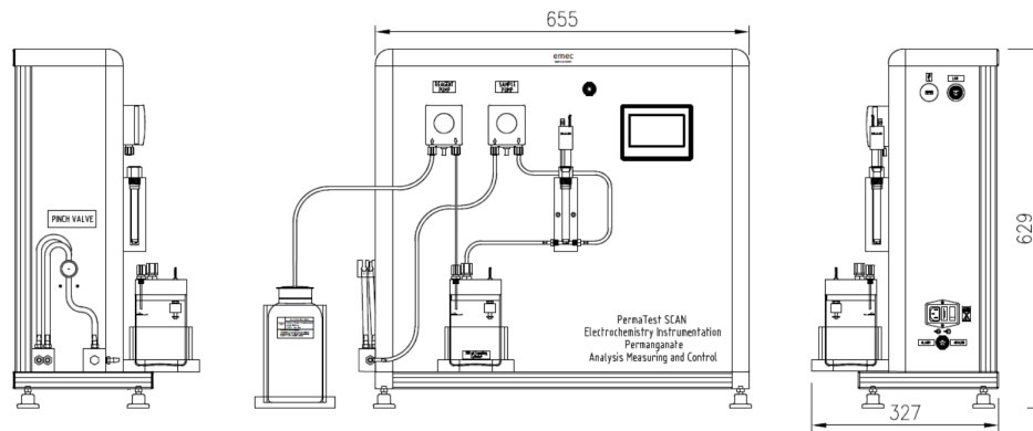
Fig. 1 - Panneau d'instrumentation
