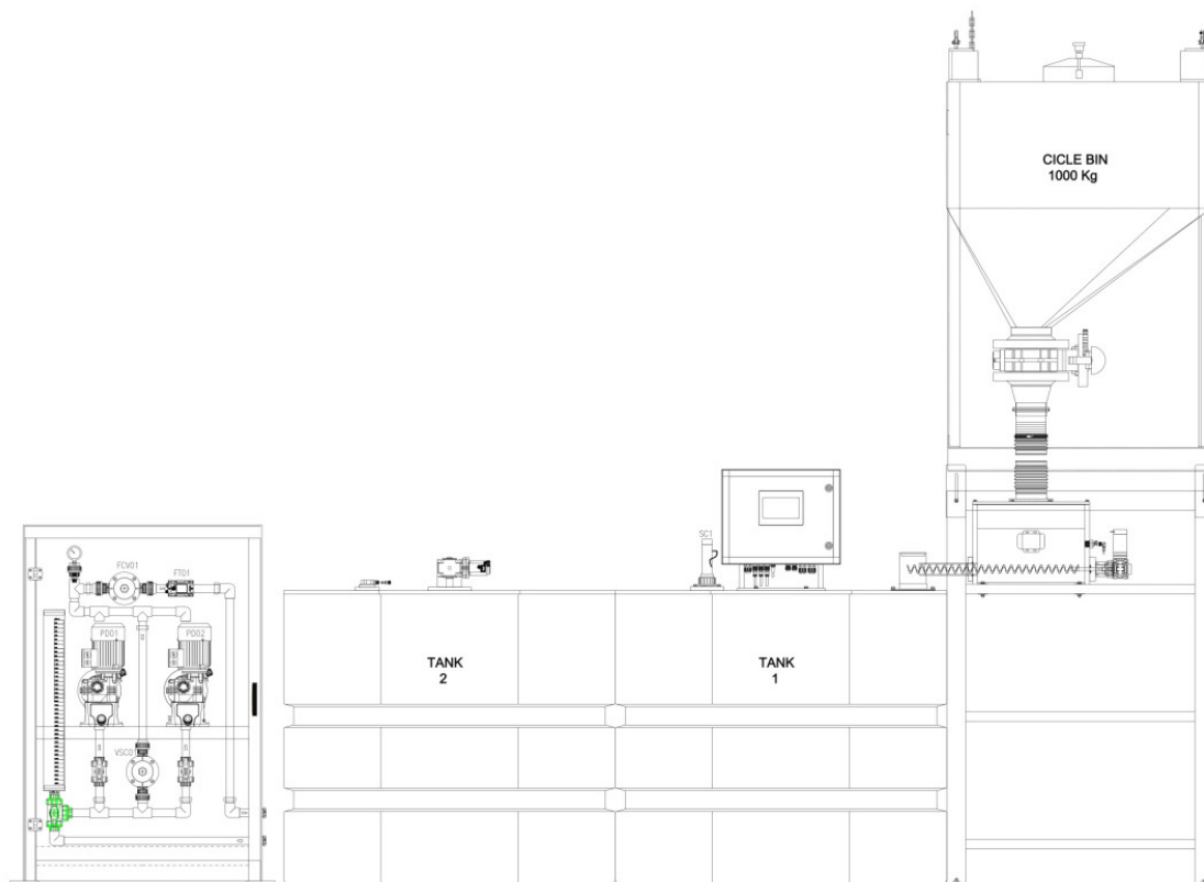
Fig. 1 - Schéma PermaDos CB + Skid Safety Box
